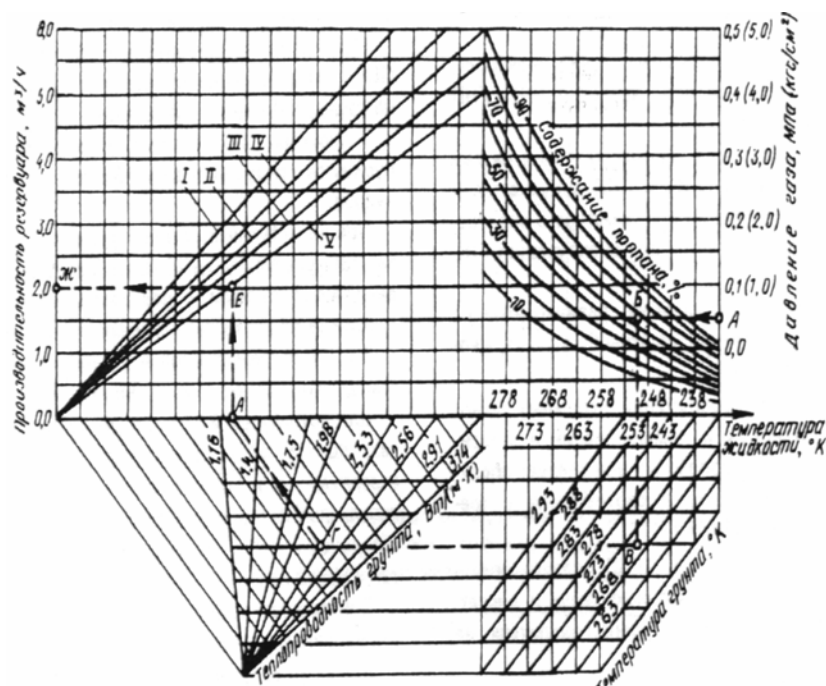
Номограмма для определения производительности резервуара сжиженного газа вместимостью 2,5 и 5 куб.м (подземного)
